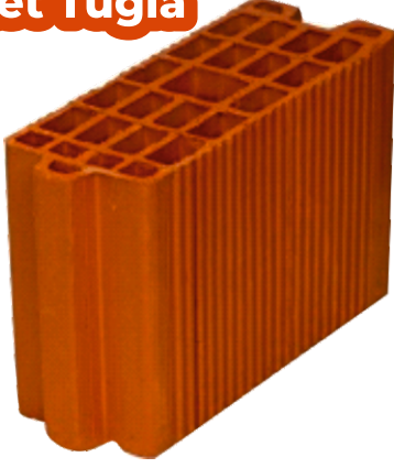
Geçmeli 29 luk Briket Tuğla
